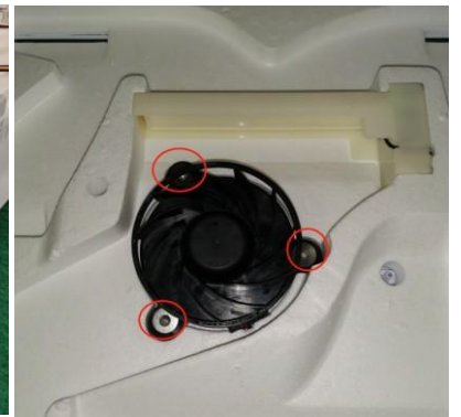
6. Removing the fan
